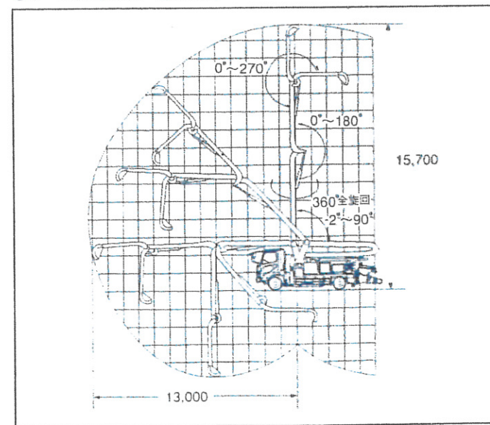
●ブーム旋回範囲図 (単位mm)
