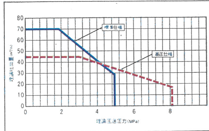
●圧送能力線図
